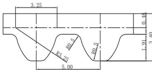
S5M带齿形
