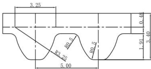
S5M带齿形
